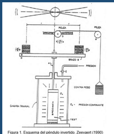
Figura 1. Esquema del péndulo invertido. Zeevaert (1990)
