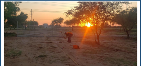
Generación de ondas elásticas mediante fuente activa (MASW). Fuente propia
